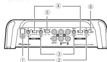
Face arrière
